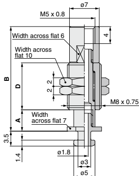
ZP3B-T2AJB■-B5
