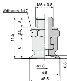
ZP3-T08UM□-A5
