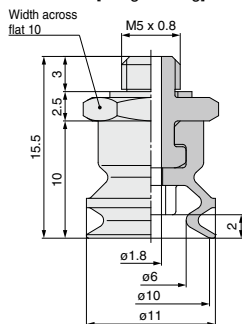
ZP3-T10B□-A5
