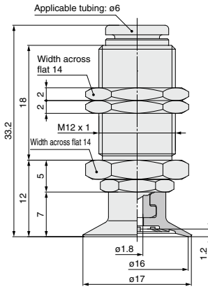
ZP3-T16UM□-A12-06
