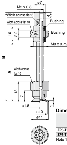
VP3-T10UM□JB■-B5
