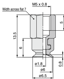
ZP3-T06UM□-B5
