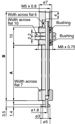
ZP3B-T2AJB■-B5
