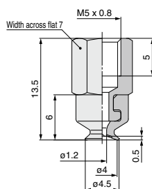
ZP3-T04UM□-B5
