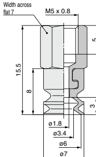
ZP3-T06B□-B5
