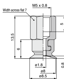
ZP3-T08UM□-B5
