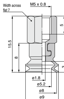
ZP3-T08B□-B5
