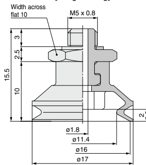
ZP3-T16B□-A5
