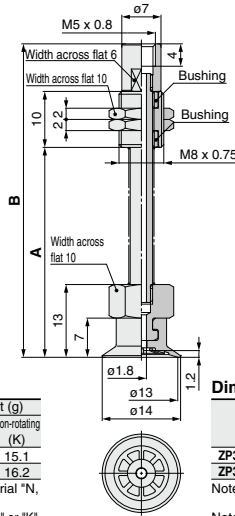
VP3-T13UM□JB■-B5
