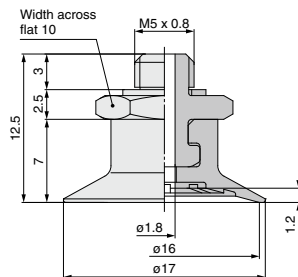
ZP3-T16UM□-A5
