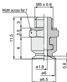
ZP3-T06UM□-A5
