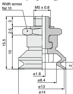
ZP3-T13B□-A5
