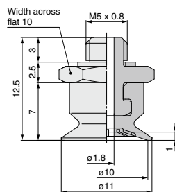
ZP3-T10UM□-A5
