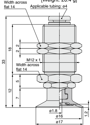
ZP3-T16UM□-A12-04
