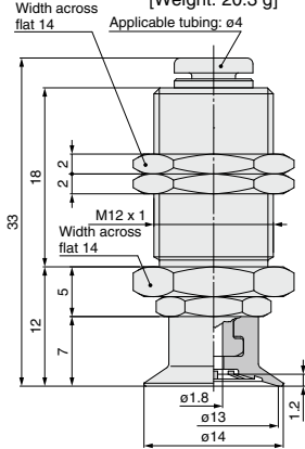
ZP3-T13UM□-A12-04
