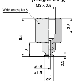
ZP3-T015U□-A6-B3
