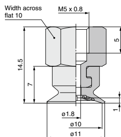
ZP3-T10UM□-B5
