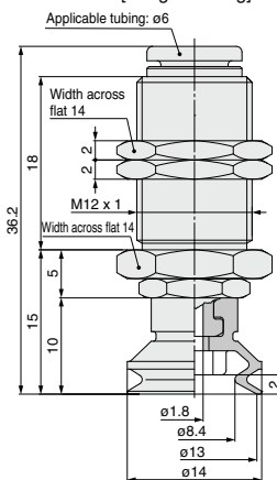
ZP3-T13B□-A12-06
