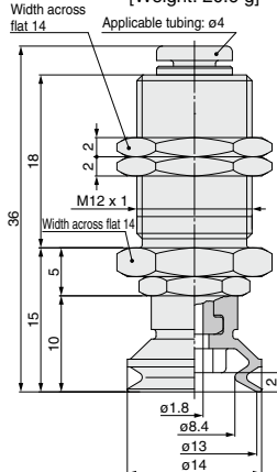
ZP3-T13B□-A12-04
