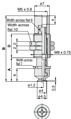
ZP3-T04UM□J■-B5
