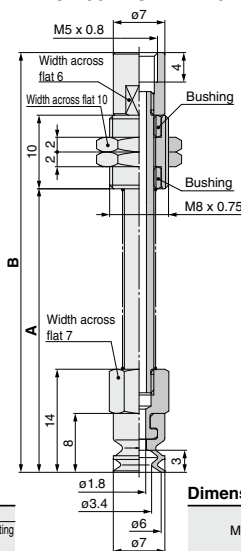
ZP3-T06B JB-B5
