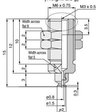
ZP3-T015U□-A6-B3
