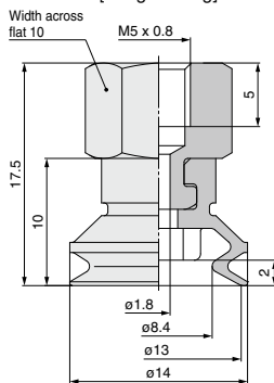
ZP3-T13B□-B5
