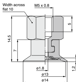
ZP3-T13UM□-B5
