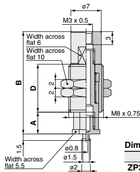
ZP3B-T1K■-B3
