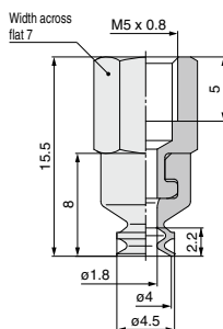
ZP3-T04B□-B5
