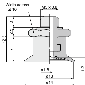
ZP3-T13UM□-A5
